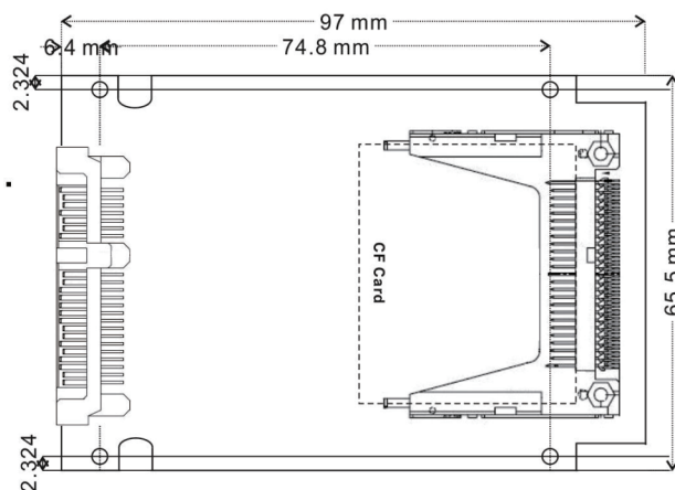
外型尺寸 (单位:mm)
